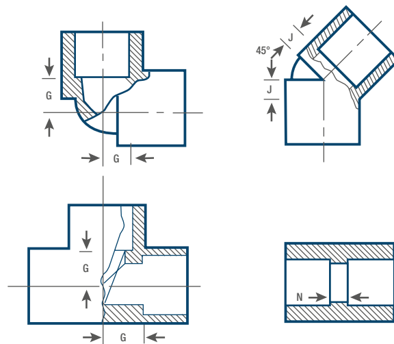
CONEXIONES ASTM F439 CPVC IPS
