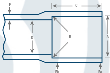
CONEXIONES ASTM D2846 CPVC CTS
