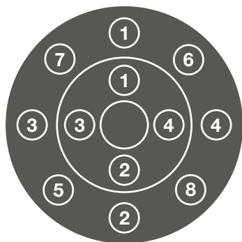
FIGURA 6. SECUENCIA DE APRIETE DE PERNOS DE BRIDA
